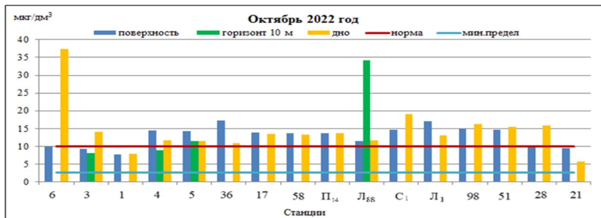
Рисунок 3.3.4. Содержание цинка в Ладожском озере в 2022 г.
