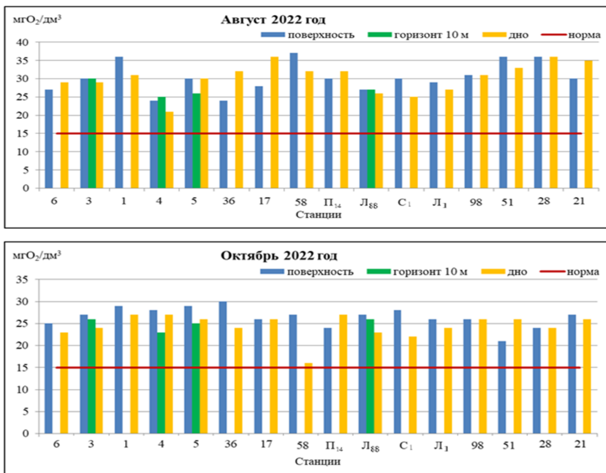
Рисунок 3.3.2. Значения ХПК в водах Ладожского озера в 2022 г.
